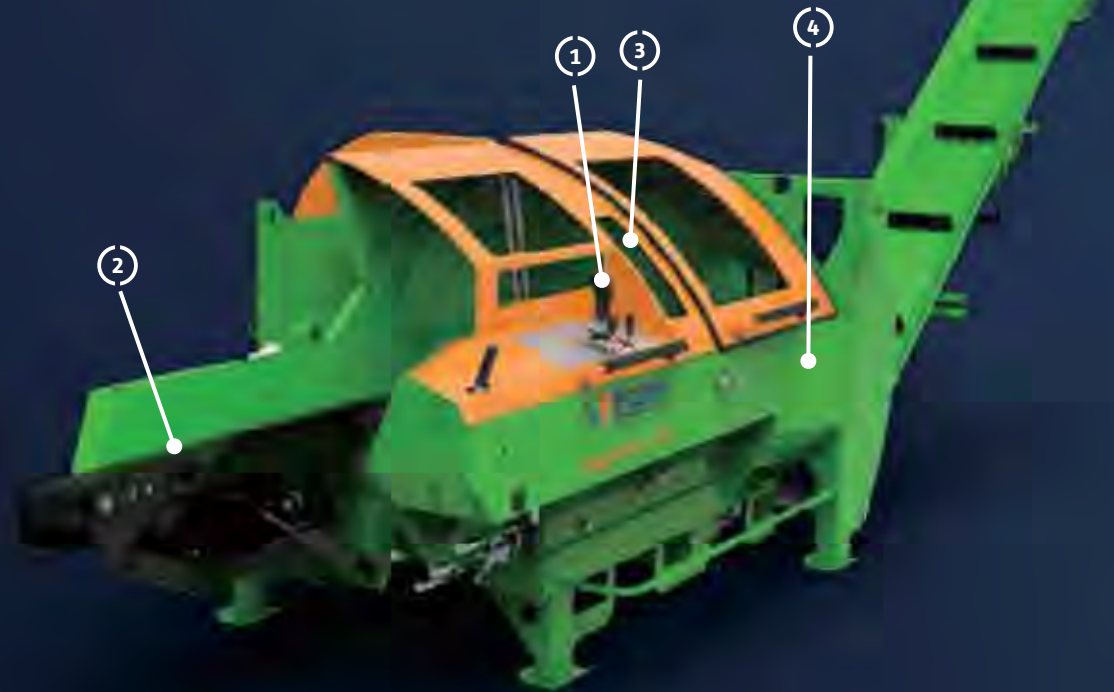
SpaltFix S-375
