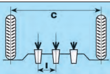
移植機のタイヤの芯～芯 条間
